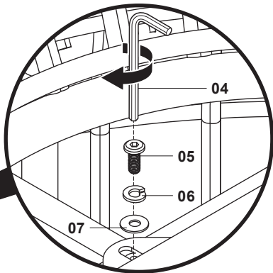
05. x8 M6 x 20 mm
