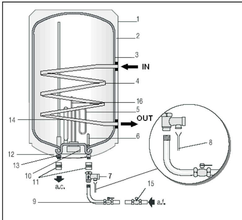
Figura 5 (Instalación vertical)
