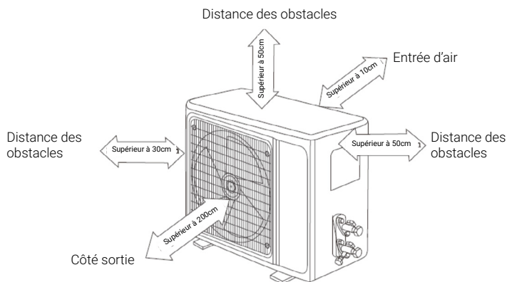
Prise en charge de l'unité extérieure
