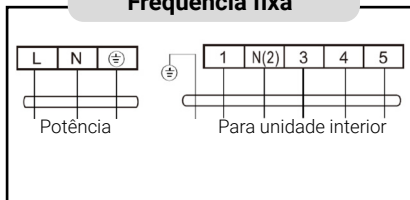
Plugue de conexão
